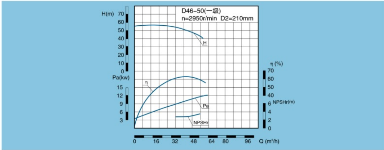
D、DG、DF、DY、DM46-50性能曲线
