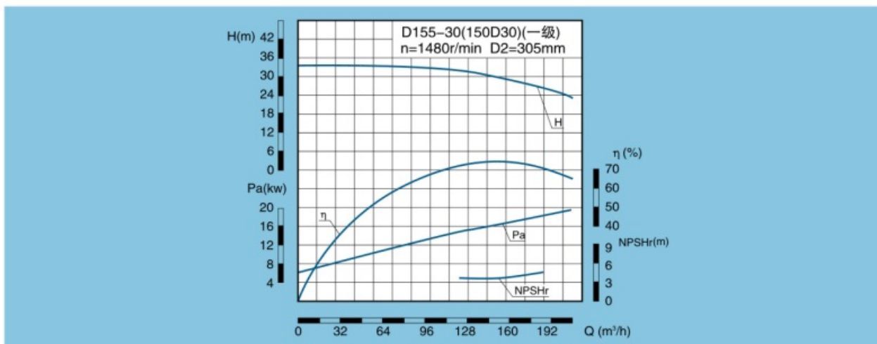
D、DG、DF、DY、DM155-30(150D30) 性能曲线 D、DG、DF、DY、DM155-30(150D30) Performance Curve
