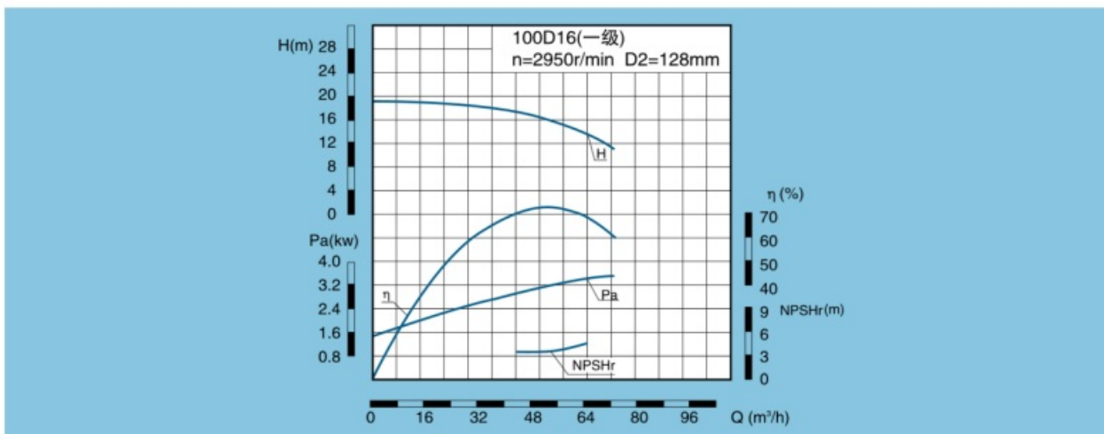
100D、DG、DF、DY、DM16 性能曲线
