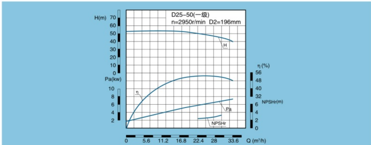
D、DG、DF、DY、DM25-50性能曲线
