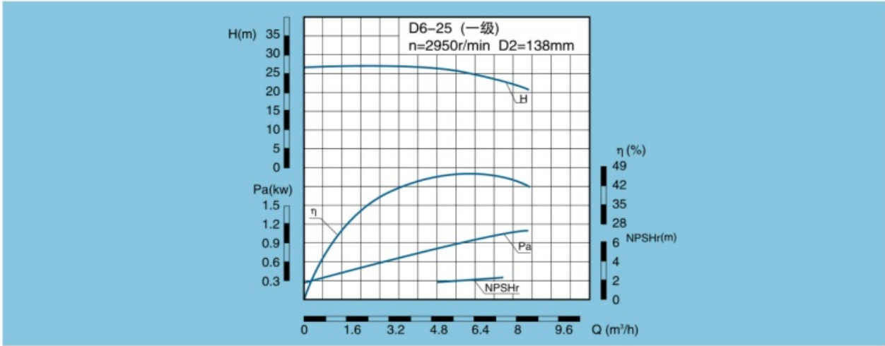
D、DG、DF、DY、DM6-25 性能曲线
