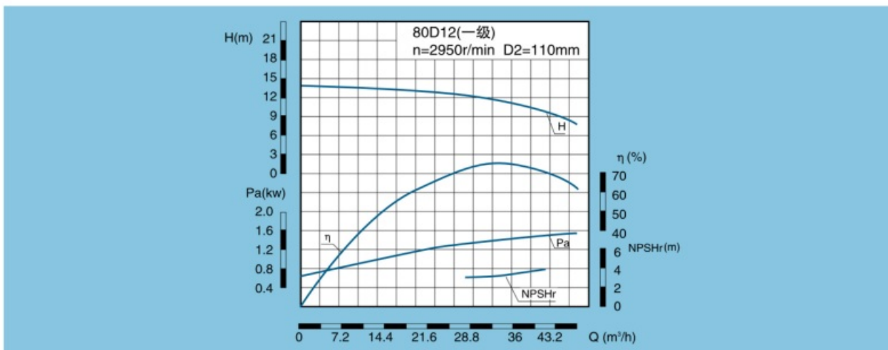
80D、DG、DF、DY、DM12 性能曲线
