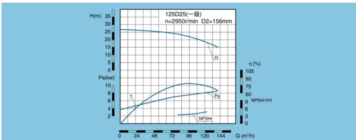
125D、DG、DF、DY、DM25 性能曲线
