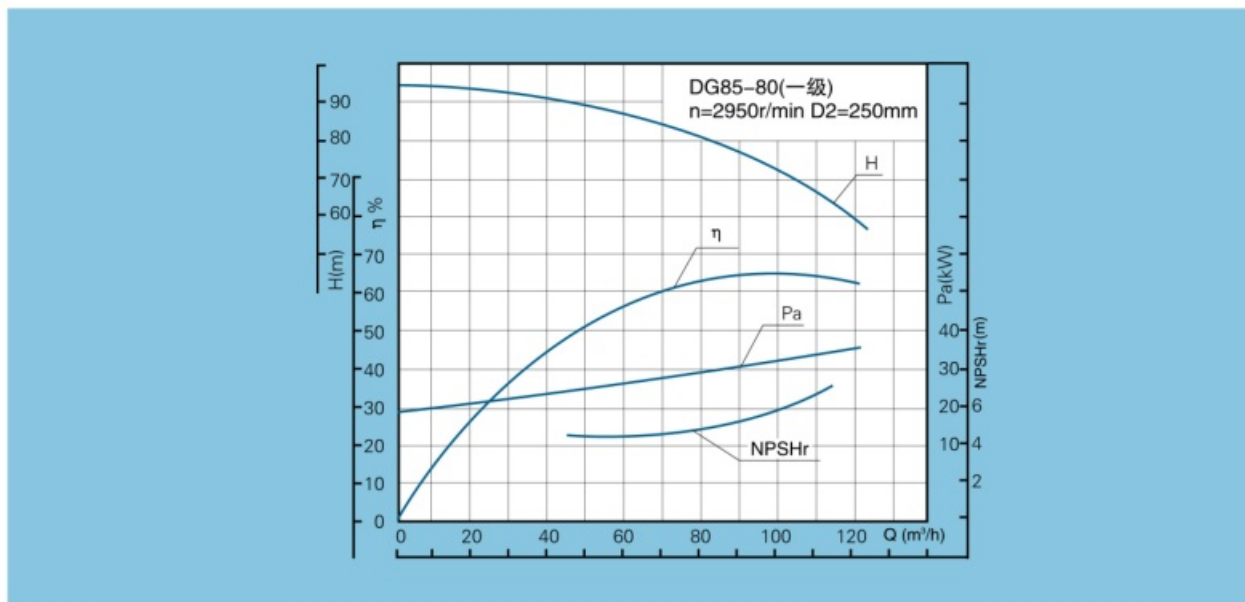
DG85-80次高压泵性能曲线表
