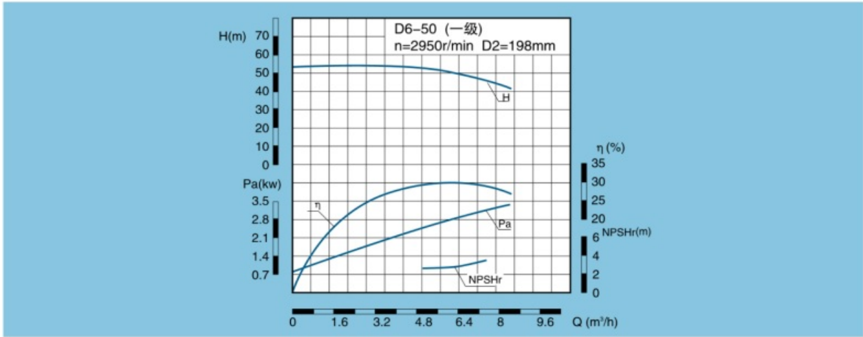
D、DG、DF、DY、DM6-50 性能曲线
