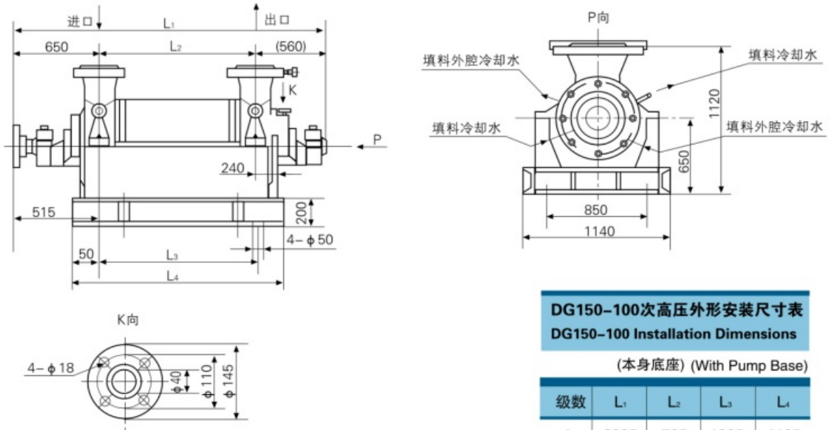
DG150-100次高压泵外形安装图
