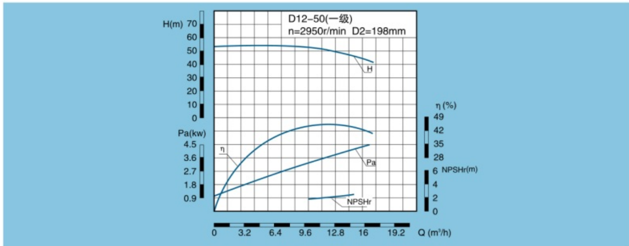
D、DG、DF、DY、DM12-50性能曲线
