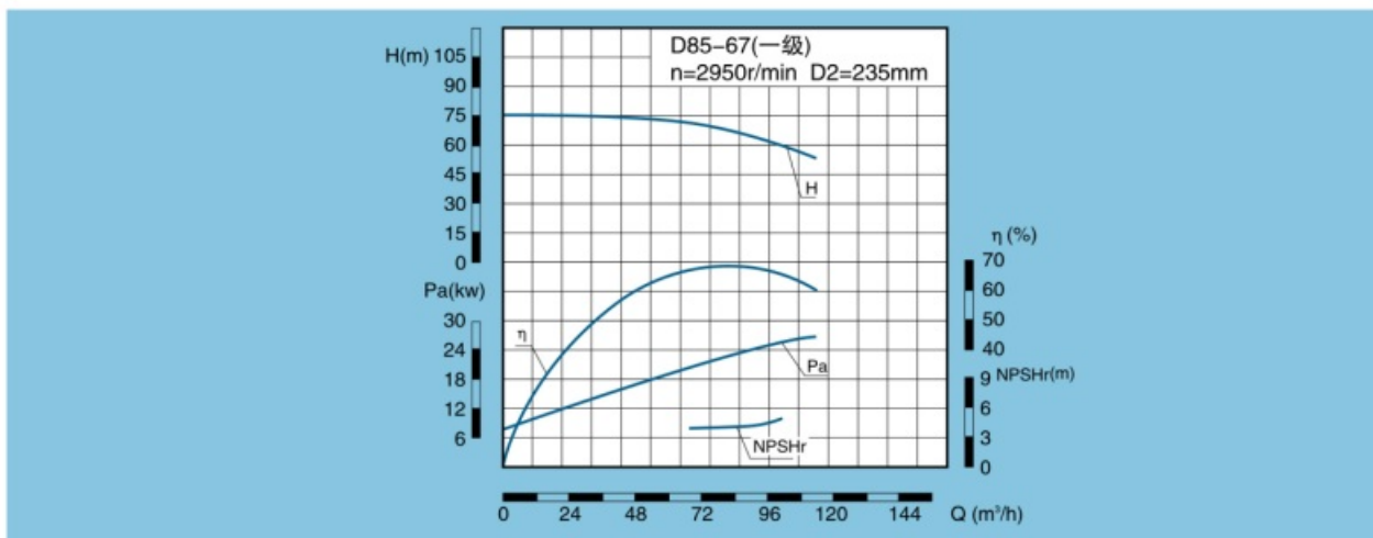
D、DG、DF、DY、DM85-67性能曲线
