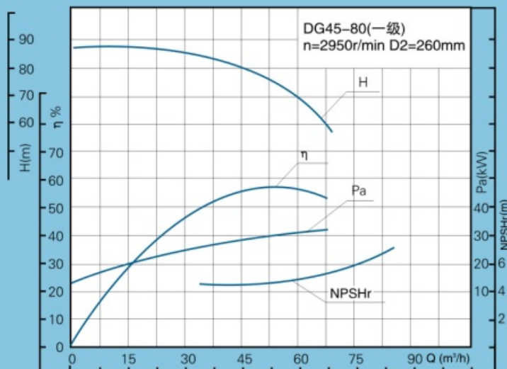
DG45-80次高压泵性能曲线表
