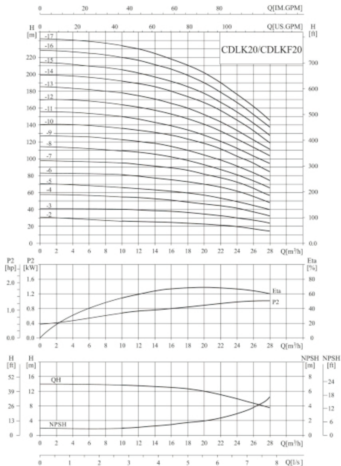
性能曲线
