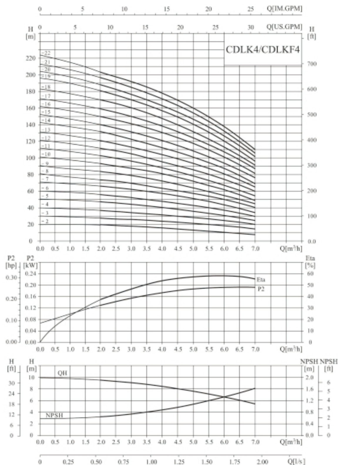
性能曲线
