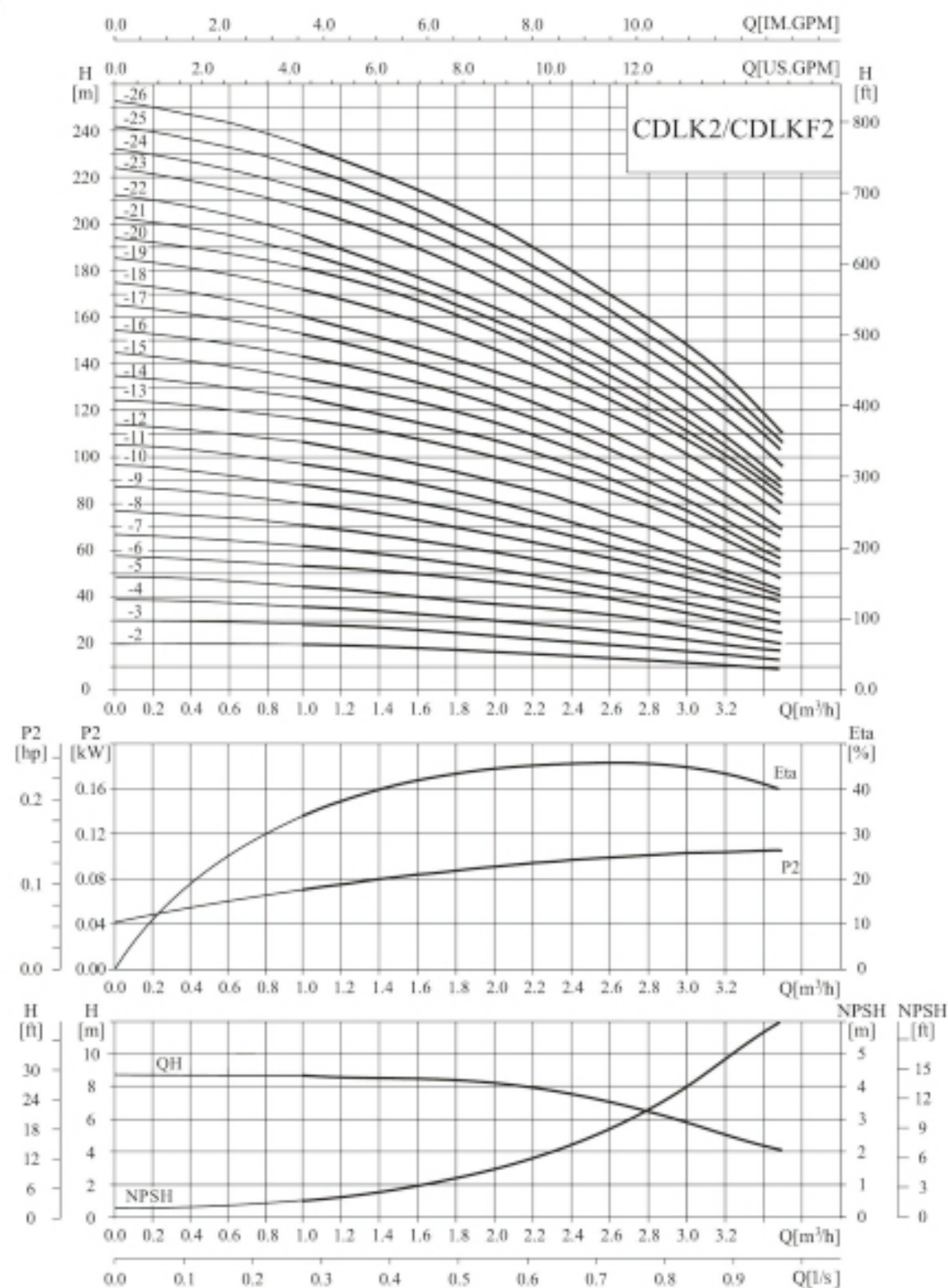
性能曲线
