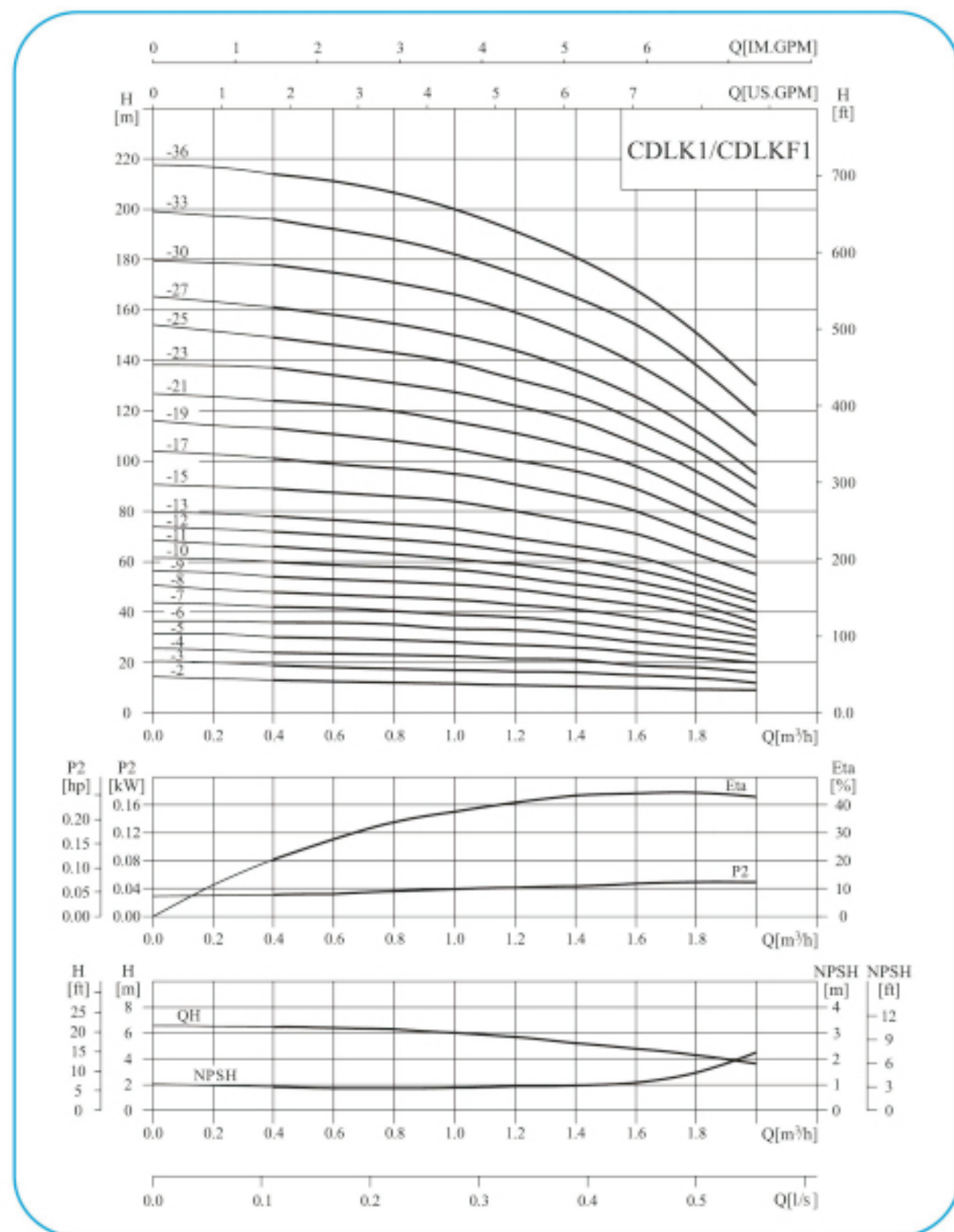
性能曲线
