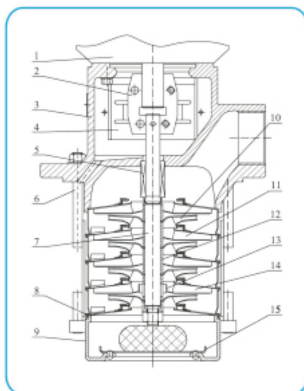
截面图 CDLK,CDLKF8,16,20
