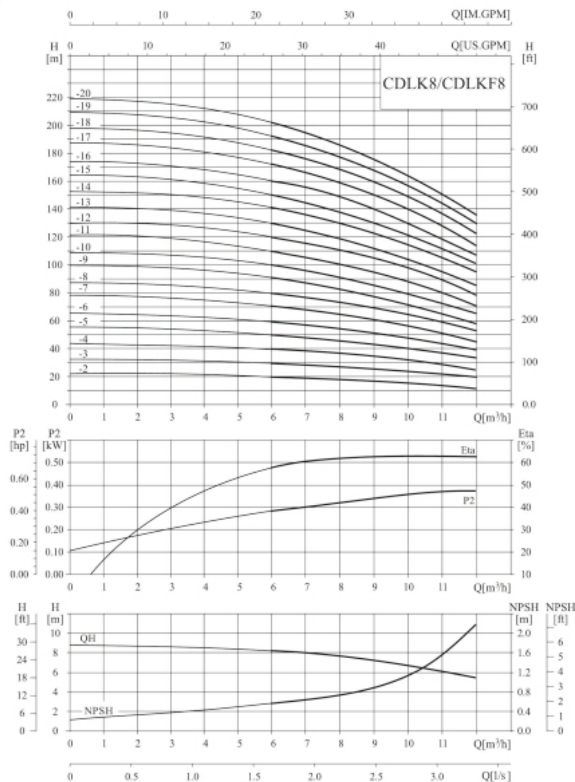
性能曲线
